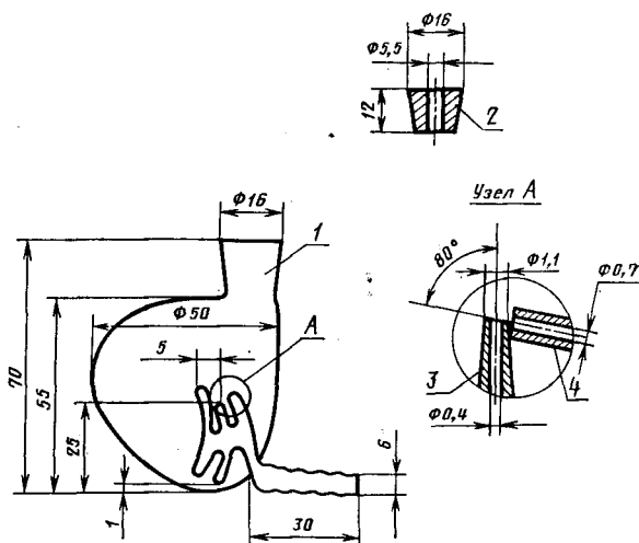
1—распылитель; 2—резиновая пробка; 3—жидкостной капилляр; 4—воздушный капилляр
